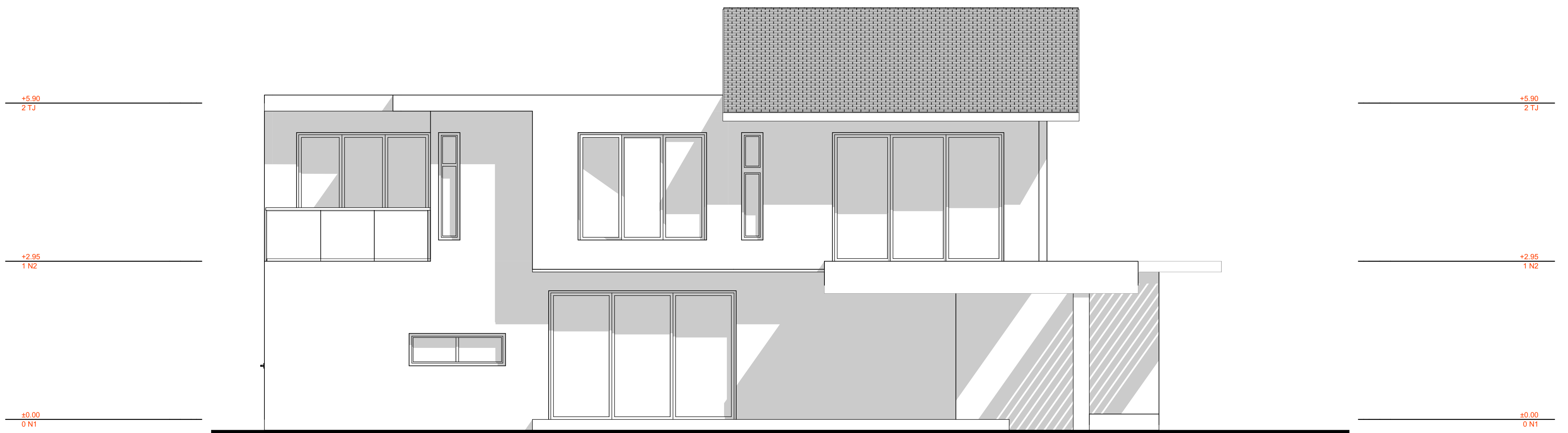
A2-EL-04 Elevacion Oeste 1:50
