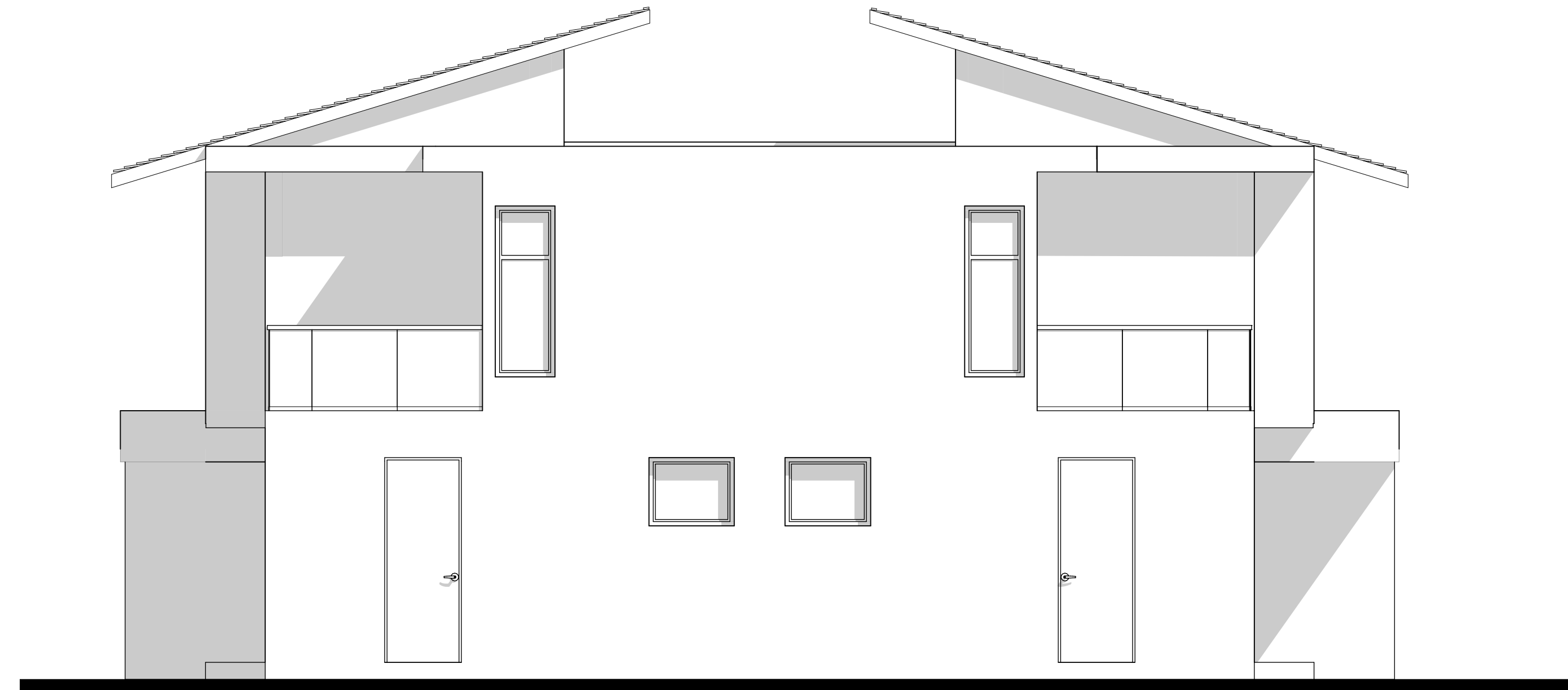
A2-EL-03 Elevacion Norte 1:50
