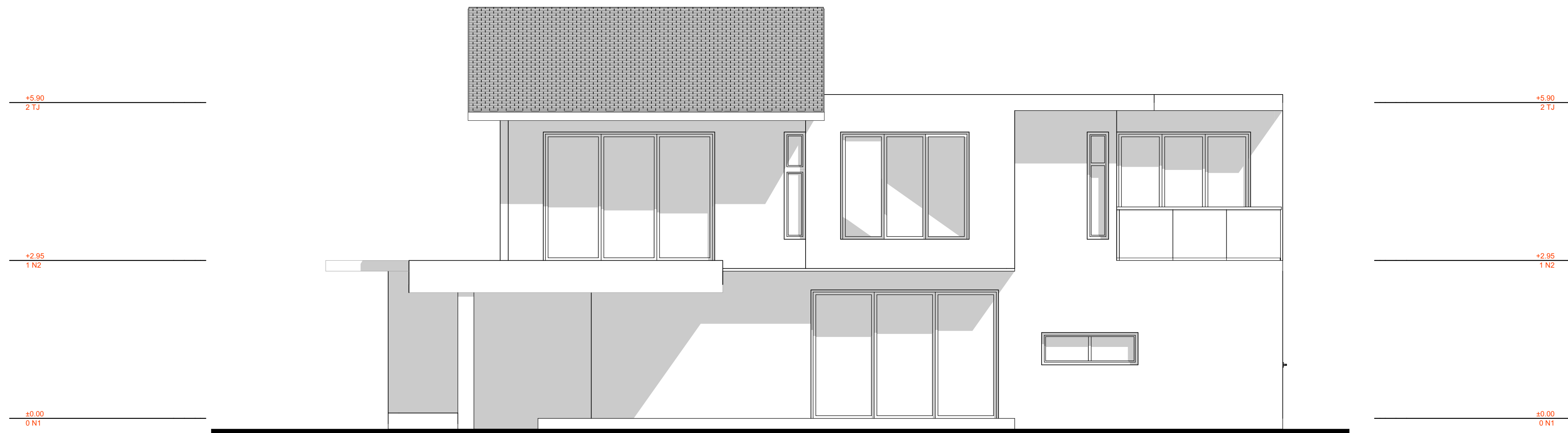
A2-EL-02 Elevacion Este 1:50
