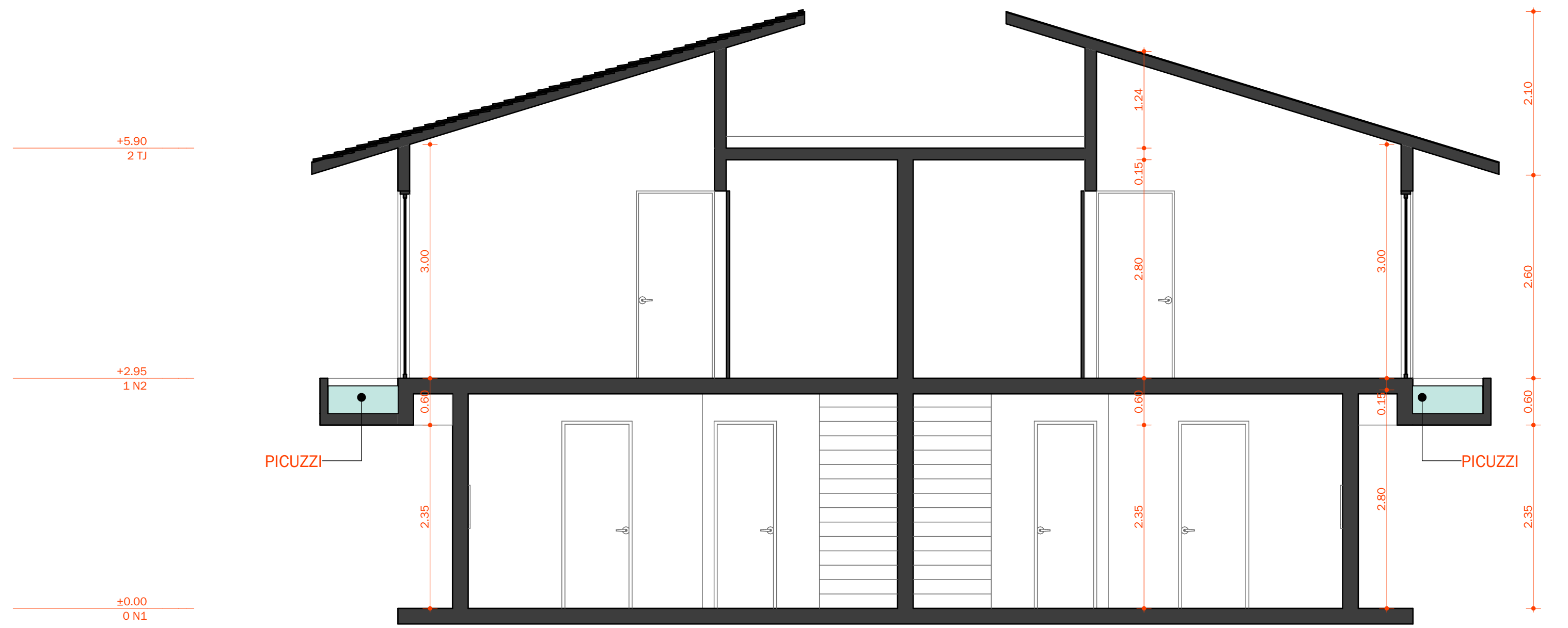
A3-SEC-01 Sección A-A' 1:50
