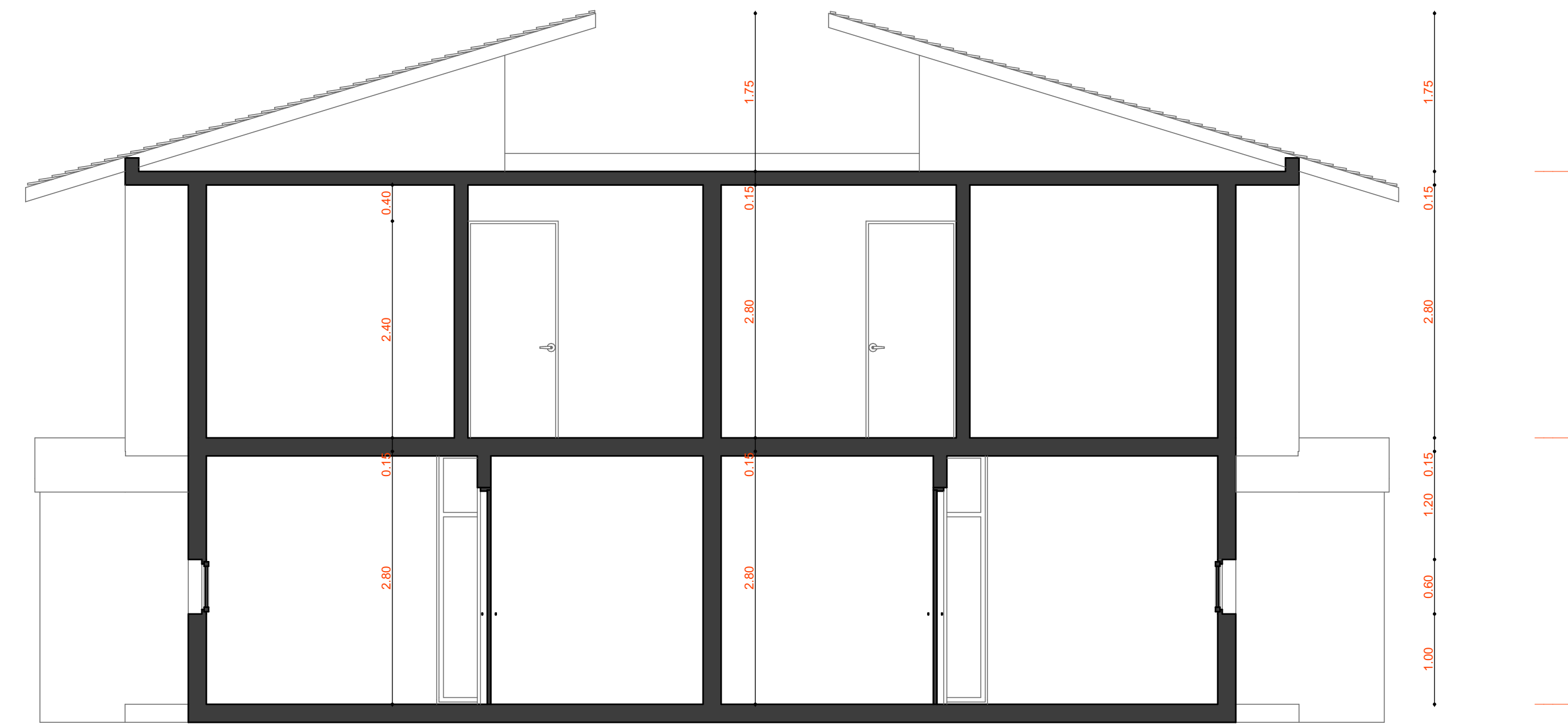
A3-SEC-03 Sección D-D' 1:50
