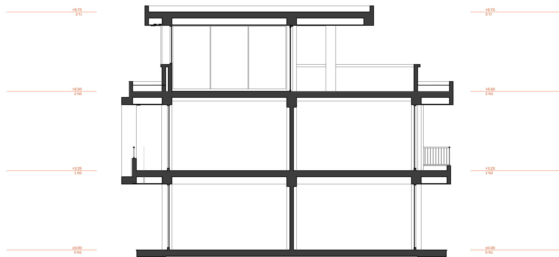
2 Sección B-B' 1:75
