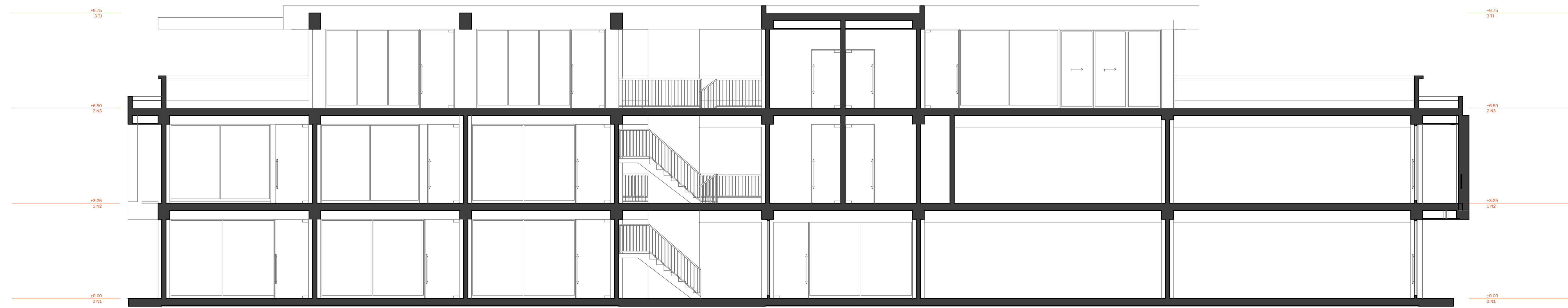
4 Sección A-A' 1:75
