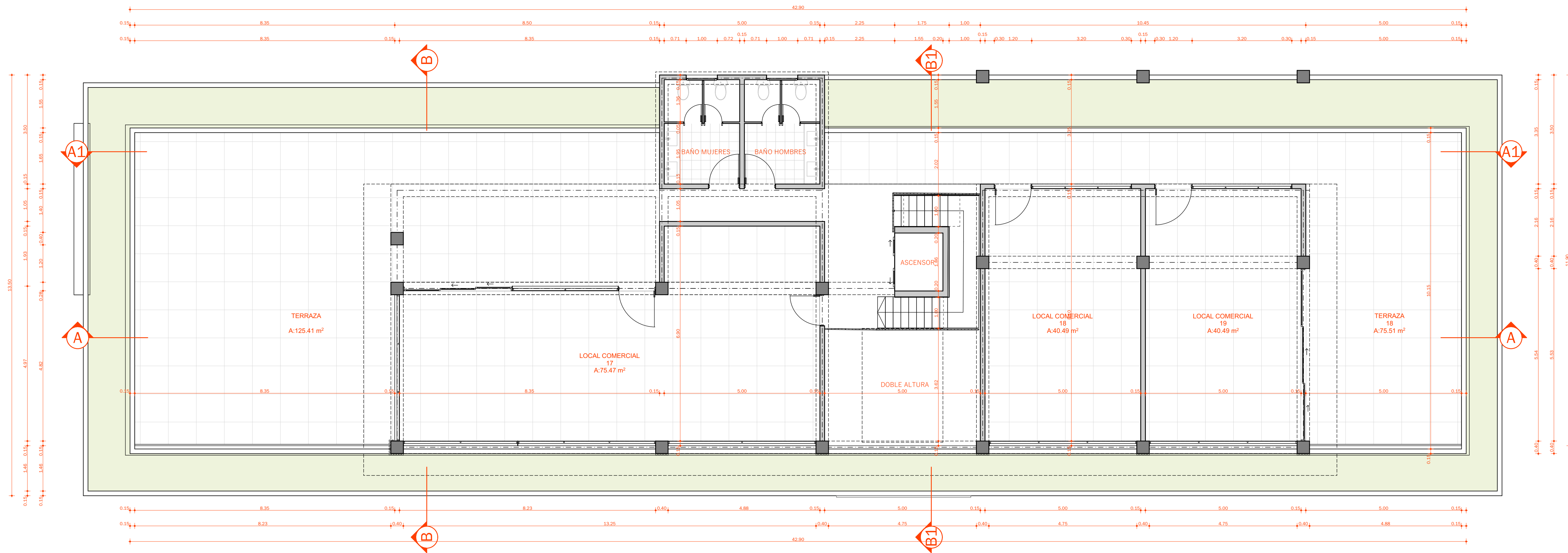
Plano Dimensionado N3
