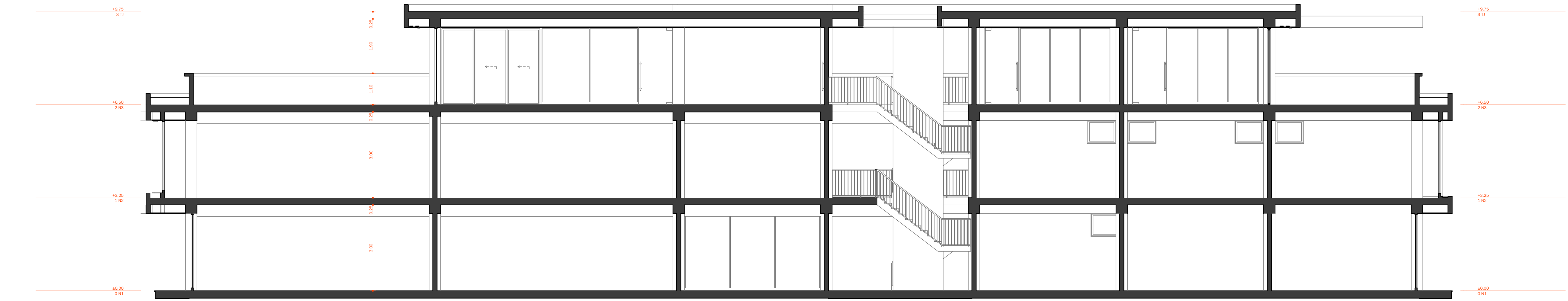
1 Sección A-A' 1:75
