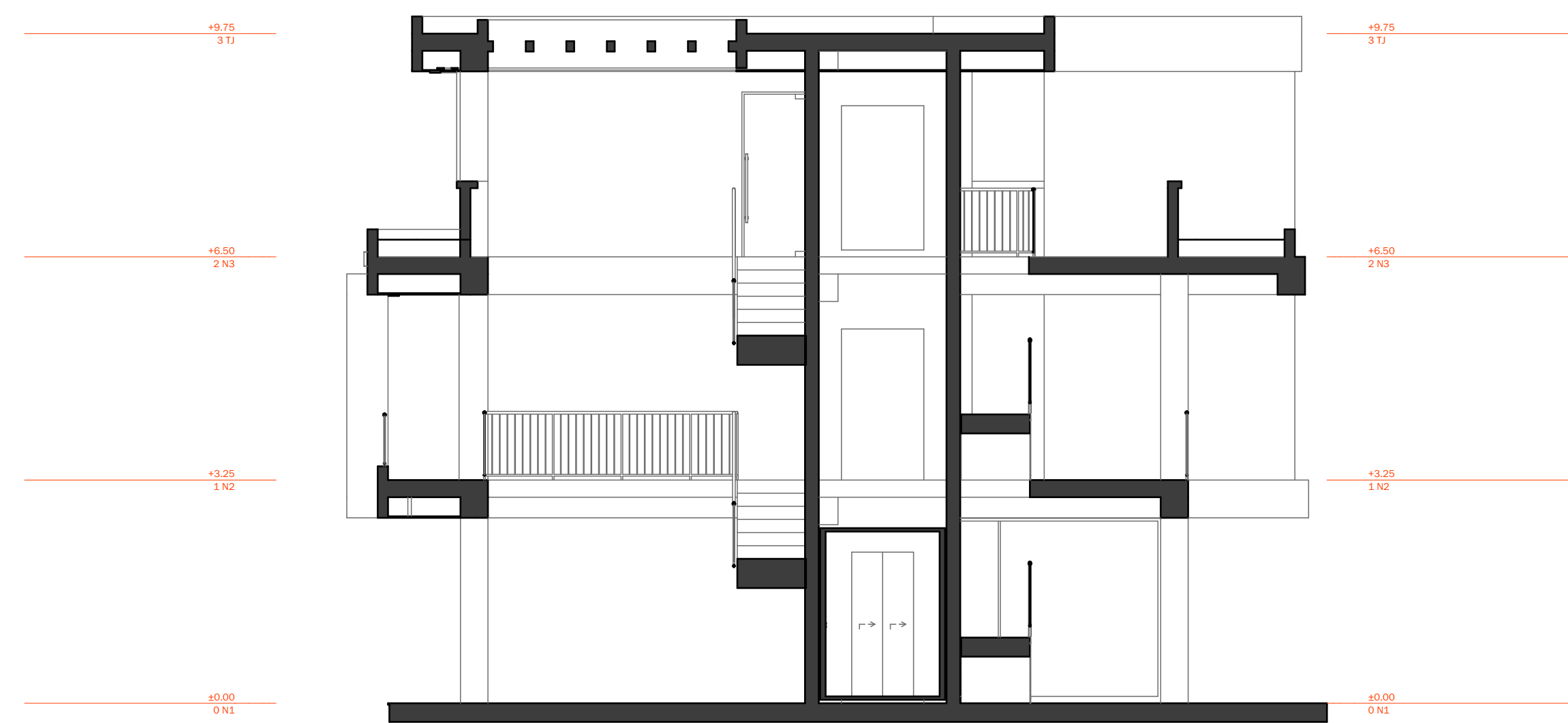
3 Sección B-B' 1:75
